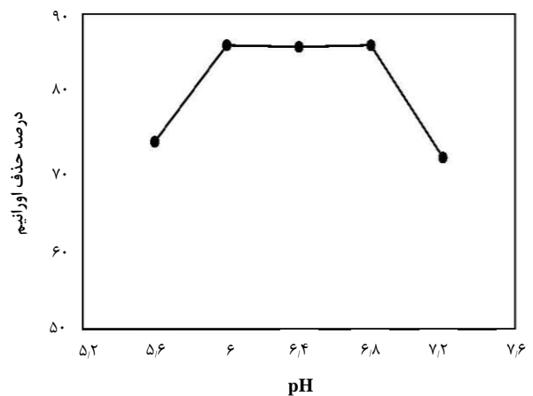
شکل ۲. درصد حذف اورانیم از محلول توسط باکتری GCWx8 در pHهای مختلف. [دما ۳۰°C، چگالی سلولی 10^9 \text{ mL}^{-1} ، مدت زمان گرمادهی ۵ روز و غلظت اورانیم ۰/۵ mM]
