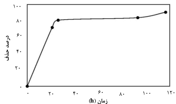
شکل ۶. سینتیک حذف اورانیم از محلول.
