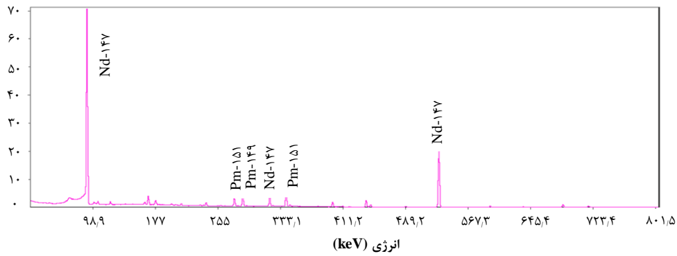
شکل ۴. طیف گامای حاصل از نمونه پرتودیده در فاصله زمانی حدود ۱۰۰ ساعت پس از پرتودهی.
