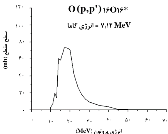
شکل ۲. سطح مقطع گسیل گاماهاى آنی ۷٫۱۲ MeV عنصر اکسیژن.
