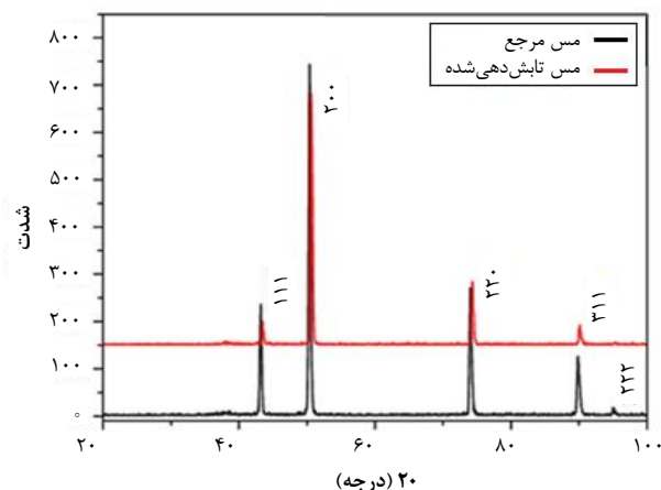
شکل ۱۰. طیف پراش پرتو ایکس نمونه‌های مس.
