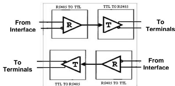
شکل ۵- نحوه بازسازی داده‌ها در گذرگاه ارتباطی برای فواصل خیلی طولانی.
