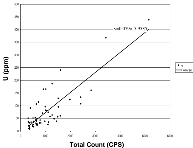
شکل ۳- نحوه ارتباط پرتوایی کل با عیار اورانیوم در ۵۵ محدوده منتخب منطقه اکتشافی خشومی.
