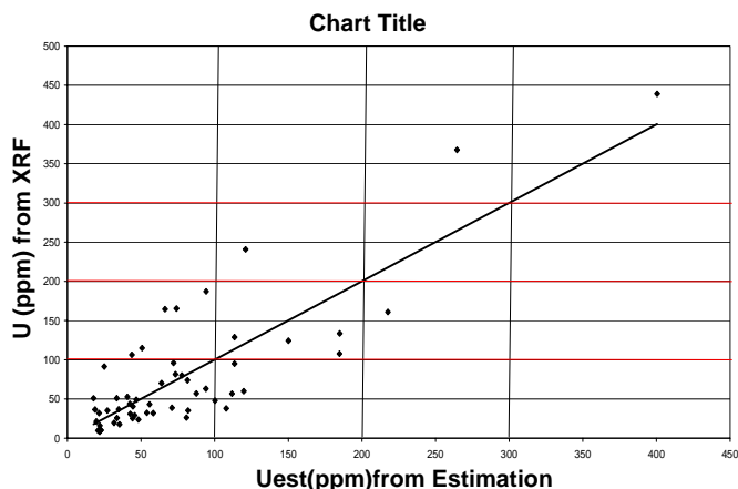
شکل ۵- نحوه ارتباط عیار تخمینی از چاه‌پیمایی و عیار حساب شده آزمایشگاهی و خط رگرسیون آن.
